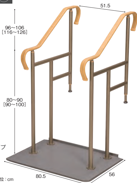
単位: cm [ ] はハイタイプの寸法です。
