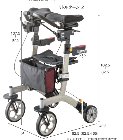
※()はZT、[]は抑速付の寸法です。
