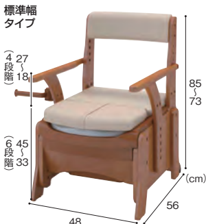
標準幅タイプ
