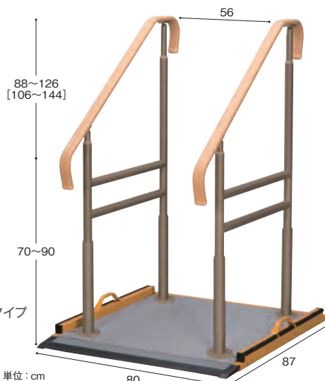
単位: cm [ ] はハイタイプの寸法です。
