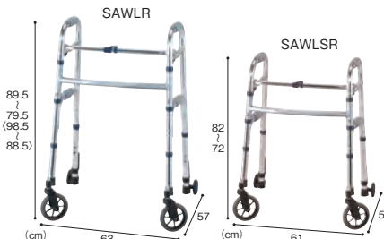
※ ( ) は SAWLHR の寸法です。
