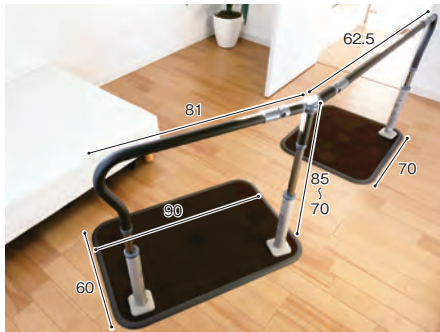
●つなぐと上下左右に角度変更可能 (※一部制約あります) 単位: cm
